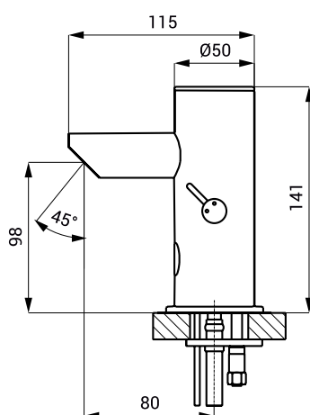
SLU 92
