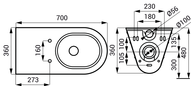
SLWN 11
