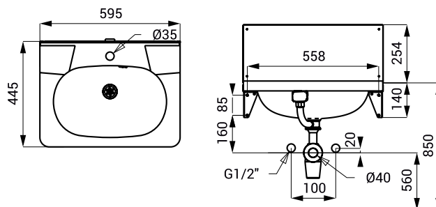
SLUN 02
