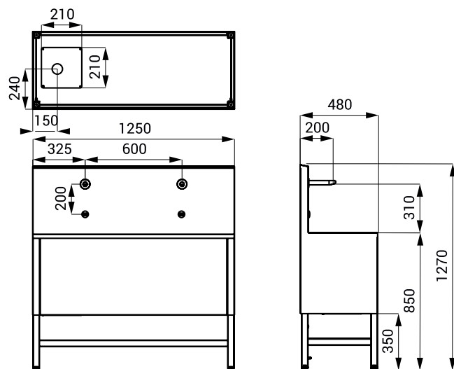
SLUN 50EA
