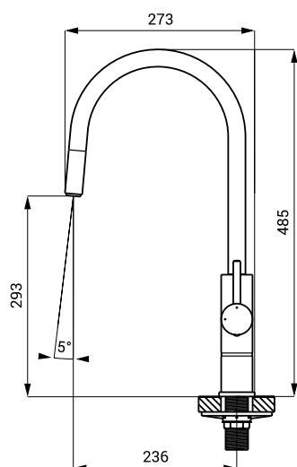
SLU 68
