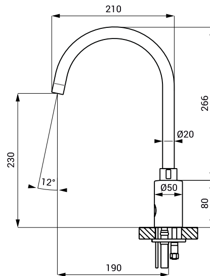
SLU 08LD
