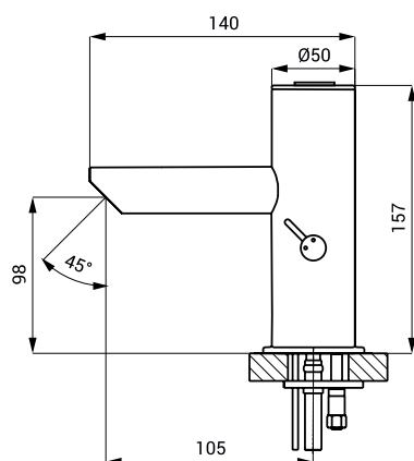
SLU 92PD
