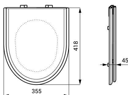
SLWN 31C
