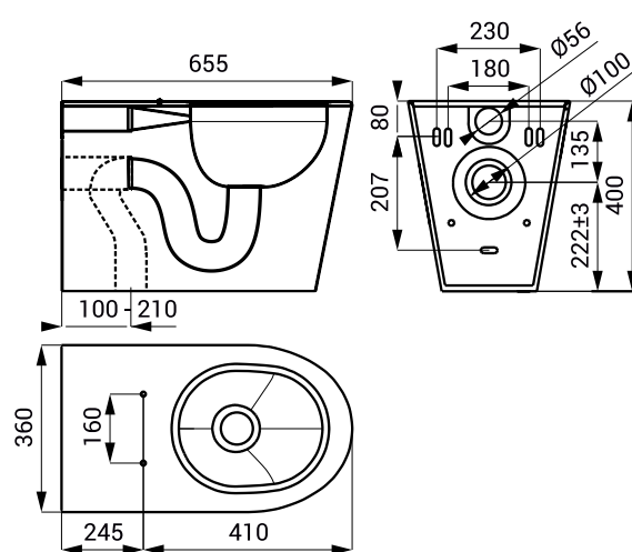
SLWN 14
