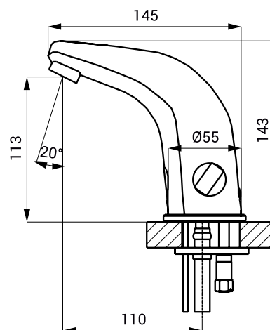
SLU 15
