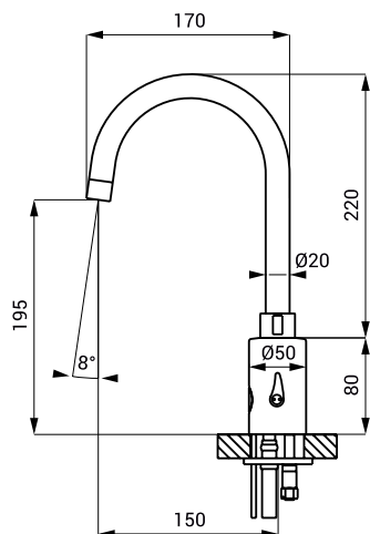
SLU 34
