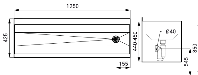
SLUN 10PA
