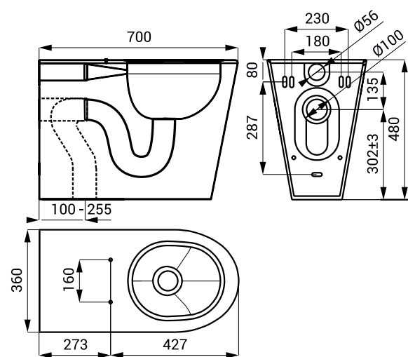
SLWN 13
